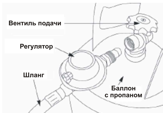
Рис 2. Подключение шланга с регулятором к газовому баллону
